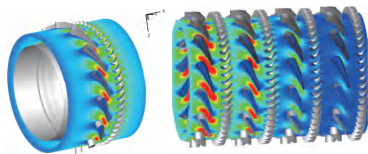
三维压气机流动模拟
