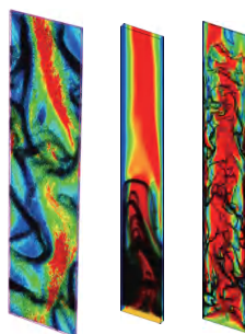
循环流化床气固两相流模拟
