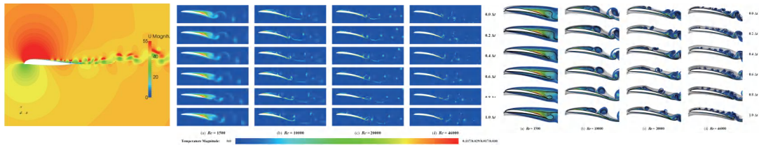
机翼转换及传热分析
