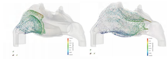
鼻腔吸入气溶胶颗粒物效果评估
