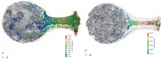
多孔介质微球捕集气溶胶病毒颗粒
