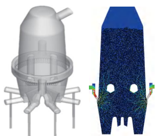
高炉炉内煤气分布模拟
