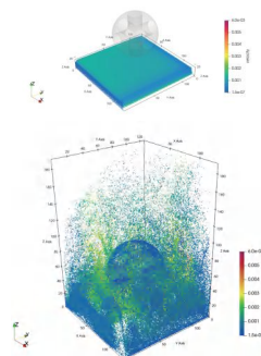
流化床内构件设计仿真
