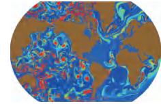
洋流湍流模拟计算
