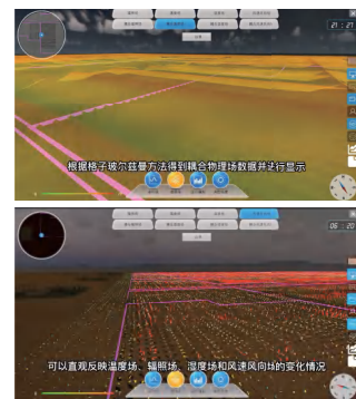
大规模光伏阵列速度、温度、湿度多物理场仿真
