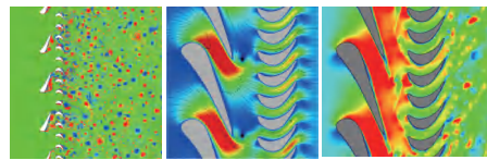
二维压气机流动模拟
